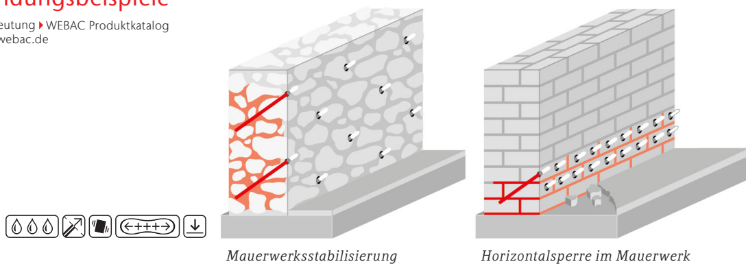
Mauerwerksstabilisierung
