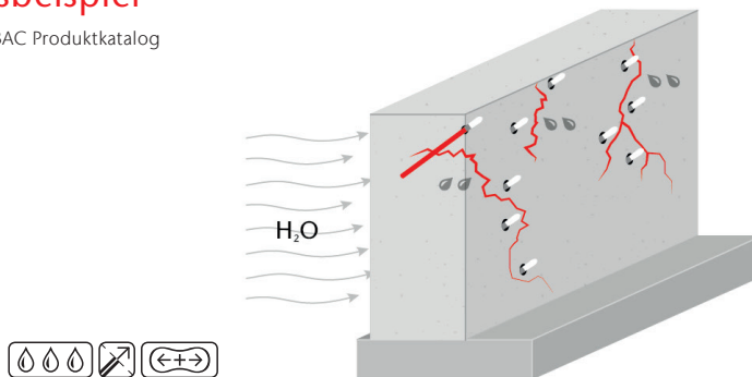
Rissinjektion in Beton bei unter Druck anstehendem Wasser
