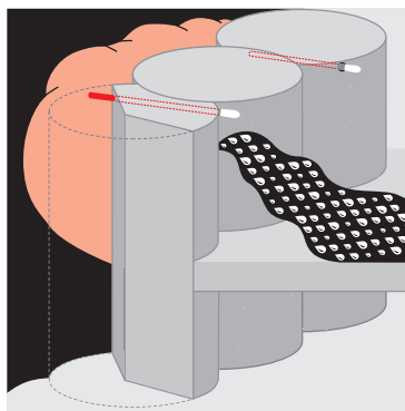
Abdichtung von Baugruben
