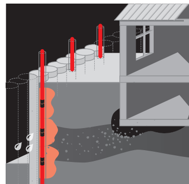
Stabilisierung und Abdichtung einer Bohrfahlwand
