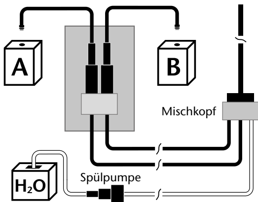
Schema einer Injektions-/Verpresseinheit
