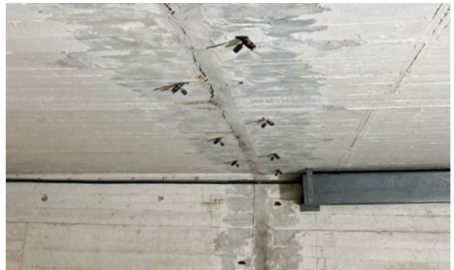
Abb. 4: Verdämmung der Fugenbereiche, Erstellen der Bohrlöcher und Setzen der Packer
