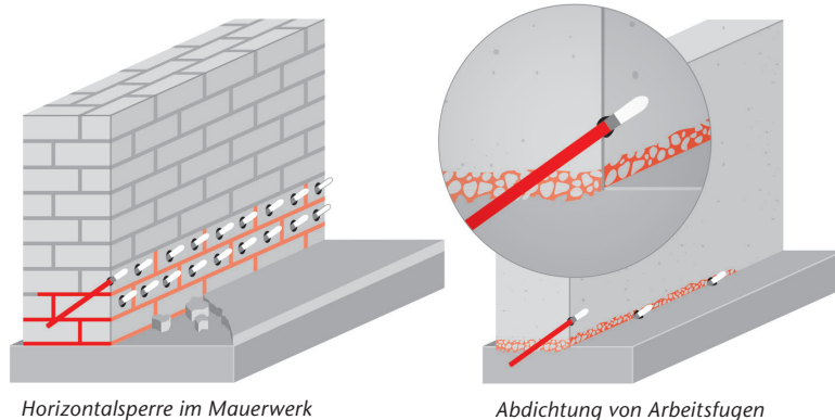
Horizontalsperre im Mauerwerk
