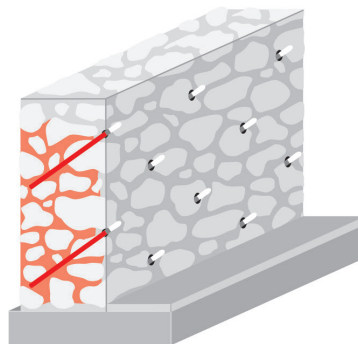
Mauerwerksstabilisierung
