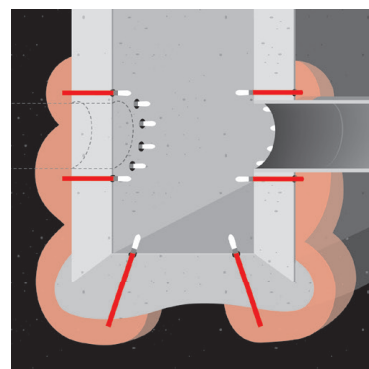
Wasserstopp- und Volumenersatzsystem bei kleineren Hohlräumen
