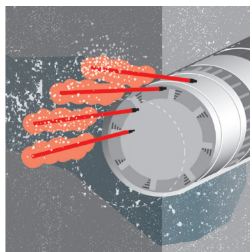
Ortsbrustverfestigung
